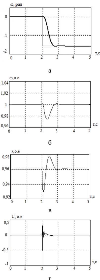
Рис.1. Результаты моделирования работы системы управления углом поворота ротора: а – отставание по углу от ведущего генератора; б – изменение частоты вращения ротора \omega ;
