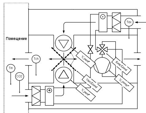
Рис.1. Функциональная схема приточно-вытяжной вентиляционной установки
