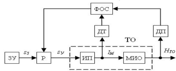
Рис.1. Блок-схема системы управления МП ТО
