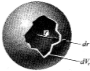
Рис.3. Радиальный заряженный слой сферы
