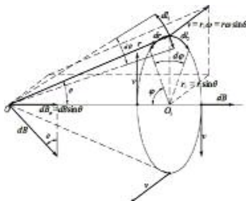
Рис.2. Расчетная схема определения магнитной индукции вращающегося шара
