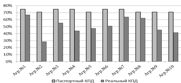
Рис.2. Паспортные и экспериментально установленные КПД насосных агрегатов
