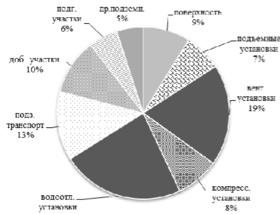
Рис.1. Распределение потребителей электроэнергии угольной шахты
