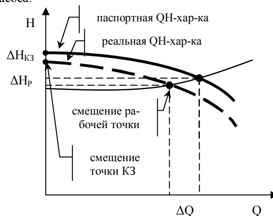
Рис.3. Смещение напорной характеристики насоса при его износе
