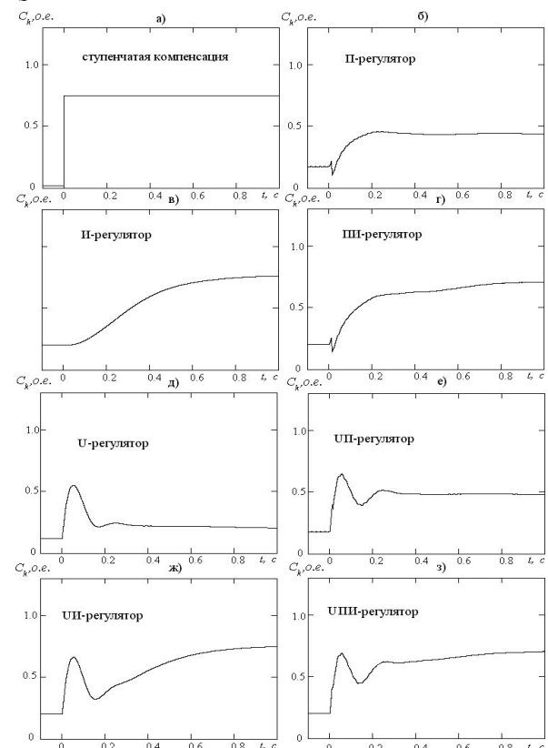
Рис. 3. Изменение емкости в системе с разными законами управления
