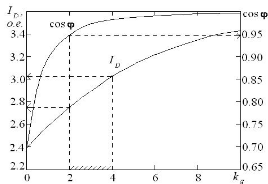
Рис.2. Зависимость величины скомпенсированного коэффициента мощности \cos \varphi и интегрального показателя качества I_D переходного процесса от настроечного параметра k_q
