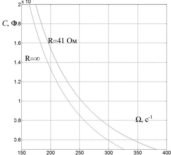
Рис.2. Зависимость емкости от частоты тока
