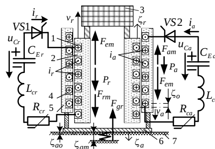
Рис.1. Схема активной электросиловой части ЛИЭД: 1, 2, 3 – обмотка, сердечник и балласт реактора; 4, 5, 6 – обмотка, сердечник и плита якоря; 7 – грунт
