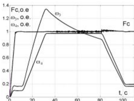
Рис.2. Переходные процессы синтезированной системы
