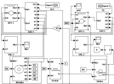
Рис.1. Модель взаимосвязанных электроприводов клетки и моталки
