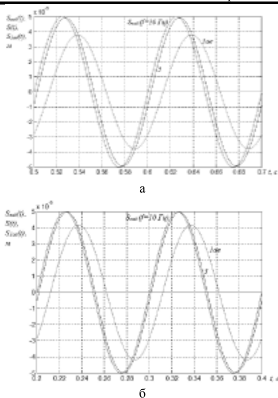
Рис. 8. Графики отработки синусоидального сигнала U_{3л.}(t) = U_{3л.М} \sin 2\pi ft ( f = 10 Гц) двухдвигательным ЭП в режиме позиционирования ( S_m = 50 мкм): а – ЭП с ЖМС; б – ЭП с СУП
