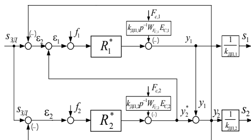
Рис.3. Обобщенная структурная схема итерационного двухдвигательного ЭП с учетом усилий нагрузки, вынесенных за контуры скорости каналов управления
