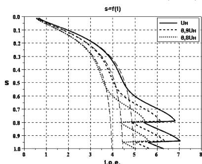
Рис.2. Ток СД при ступенчатом изменении значения емкости накопителя C = 75; 100; 150 мкФ
