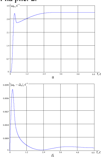
Рис.2. Реальна швидкість обертання ротора (а) та помилка у визначенні швидкості за допомогою спостерігача Люенбергера (б)
