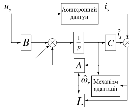
Рис.1. Структура спостерігача Люенбергера Математична модель асинхронного двигуна може бути записана так:
