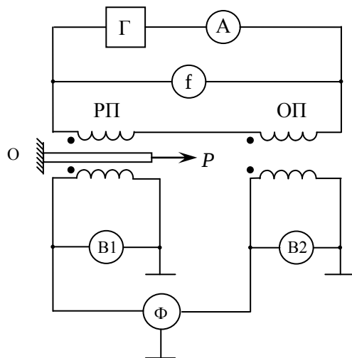
Рис. 1. Схема установки, реализующей амплитудно-частотный и фазово-частотный методы
