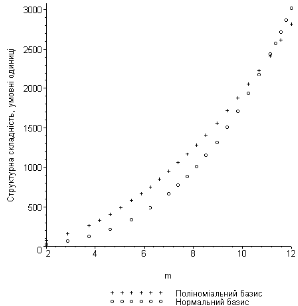
Рис. 9. Структурна складність помножувачів для поліноміального та нормального базисів ( m < 12 )
