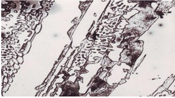
Рис. 2. Мікроструктура литих Fe-C-V сплавів. Швидкість охолодження при кристалізації а, в, д, ж, з – 60 град/мин, б, г, є – 400 град/мин.
