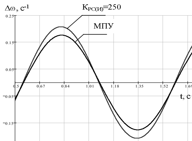
Рис.4. Динамическая ошибка систем при обработке синусоидального задания на скорость
