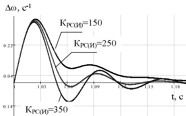
Рис.2. Динамическая ошибка релейной системы в результате наброса нагрузки при разных K_{PC(i)}
