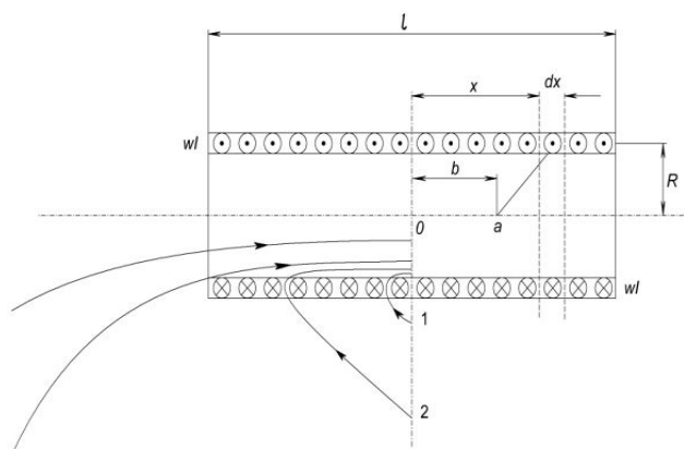
Рис. 2. Магнитное поле соленоида
