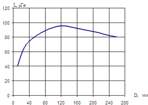
Рис.4. Зависимость L = f(D) при длине провода l=10 \text{ м}
