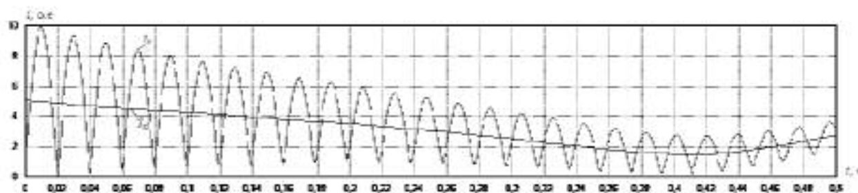
Рис. 3. Выделение периодической составляющей тока К3
