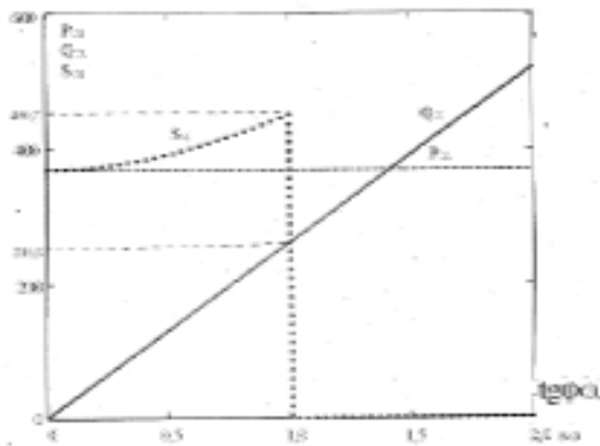
Рис. 4. Залежність навантаження синхронного двигуна за умови \beta_{СД} = 0,92
