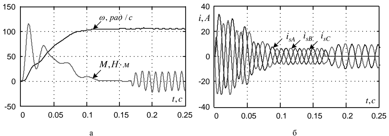
Рис. 2. Переходные процессы при прямом пуске АД и обрыве фазы С статора на установившейся скорости без нулевого провода: электромагнитный момент и скорость вращения (а), токи статора (б)
