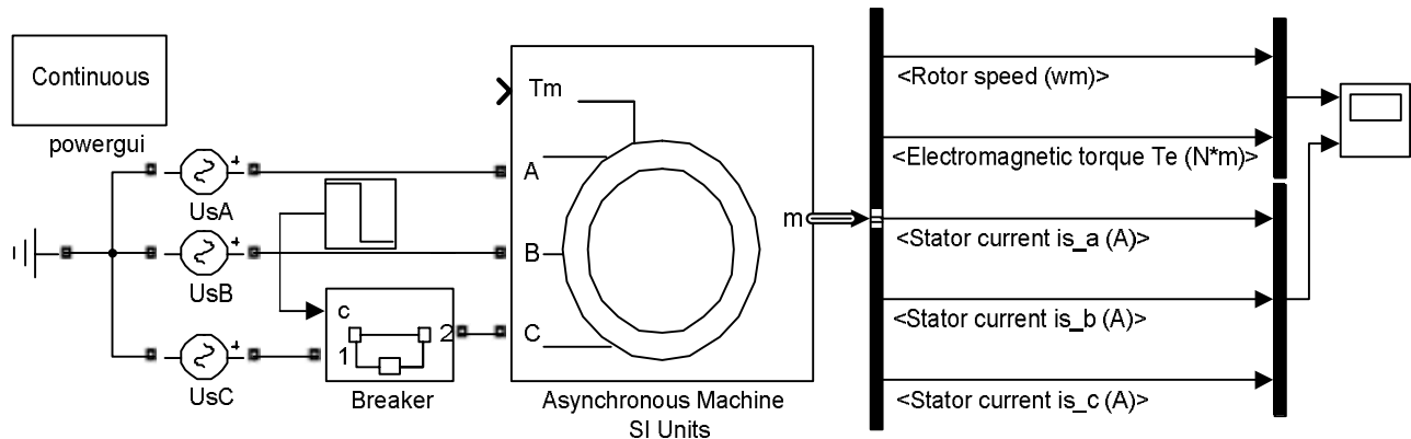
Рис. 1. Модель для исследования обрыва фазы статора асинхронного двигателя с использованием блока Asynchronous Machine SI Units
