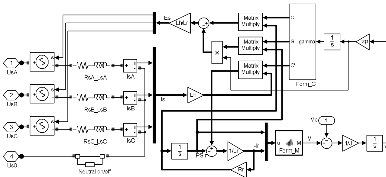
Рис. 5. Схематехническая модель асинхронного двигателя
