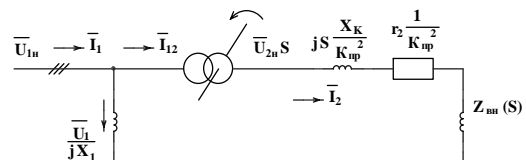
Рис. 2. Схема замещения двигателя в форме вращающегося трансформатора
