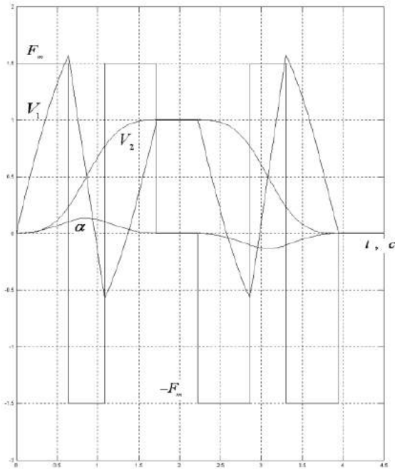
Рис. 2. Графік оптимального перехідного процесу пуску та гальмування механізму горизонтального переміщення
