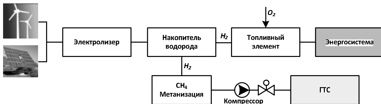
Рис. 1. Структурная схема получения и преобразования водорода
