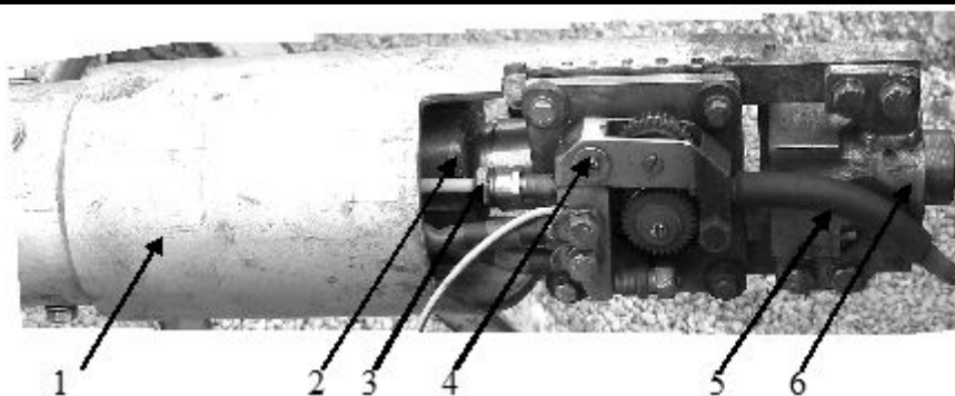
Рис. 1. Автомат для сварки в стеснённых условиях на большой глубине: 1 – корпус; 2 – механизм вращения; 3 – направляющий канал; 4 – подающий механизм с колебателем мундштука; 5 – мундштук; 6 – крепление и элементы токопередачи на доньшко
