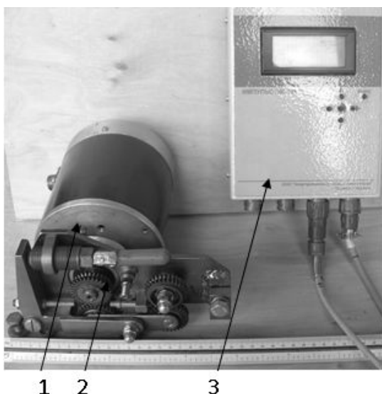
Рис. 2. Механизм подачи электродной проволоки на основе вентильного электропривода: 1 – электродвигатель; 2 – прижимной узел; 3 – компьютеризованный блок управления
