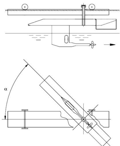
Рис. 1. Экспериментальная установка для изучения работы гребного винта в косом потоке
