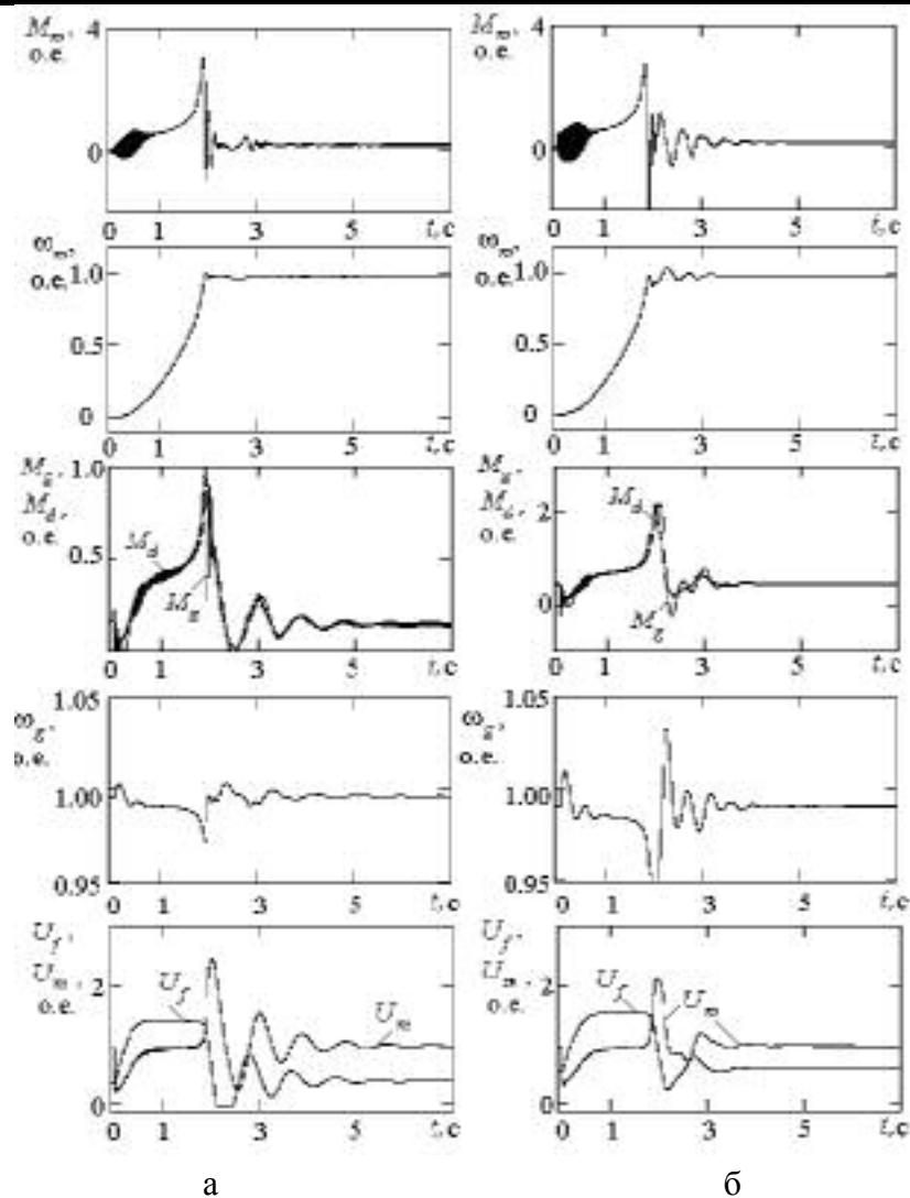
Рис. 1. Переходные процессы пуска асинхронного электродвигателя мощностью 20 % от номинальной мощности дизельного электроагрегата с синхронным генератором при начальной нагрузке дизель-генератора в 12,5 % (а) и 50 % (б)
