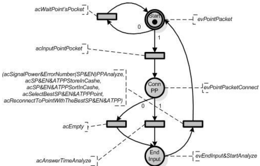
Рис. 2. Сети Петри внутреннего роуминга Wi-Fi
