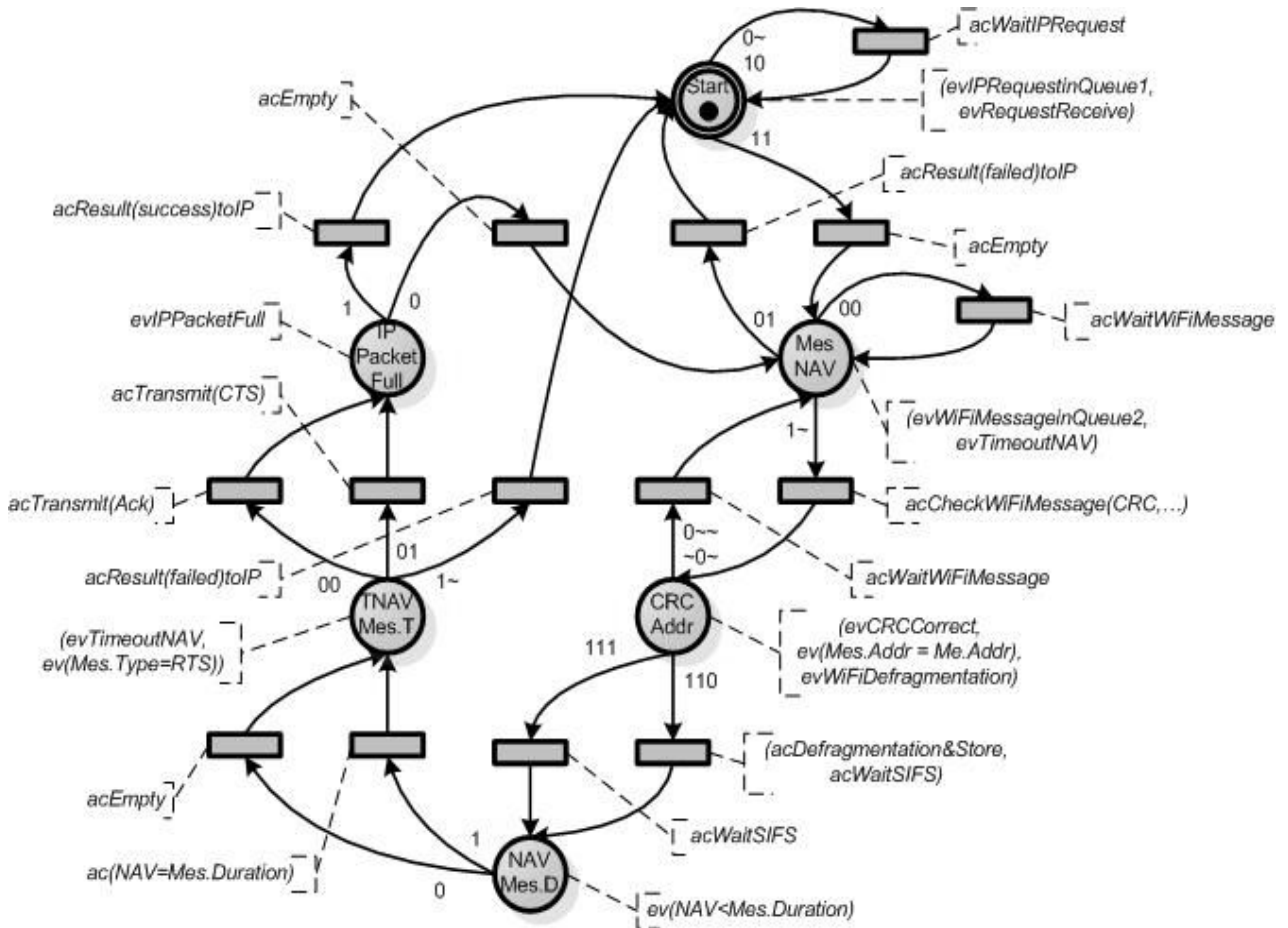
Рис. 1. Сети Петри приемника Wi-Fi
