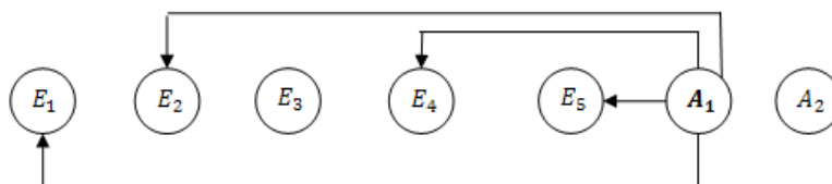
Рис. 6. Граф для индикатора A_1
