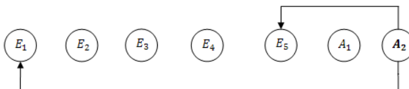
Рис. 7. Граф для индикатора A_2
