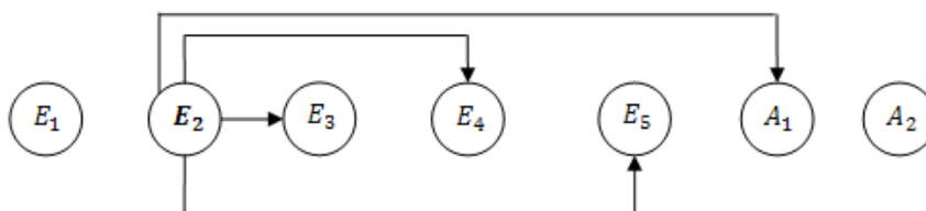
Рис. 2. Граф для индикатора E_2
