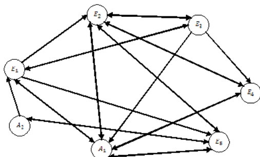
Рис. 8. Ориентированный граф для всех индикаторов ценности
