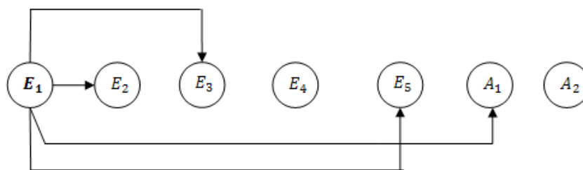
Рис. 1. Граф для индикатора E_1
