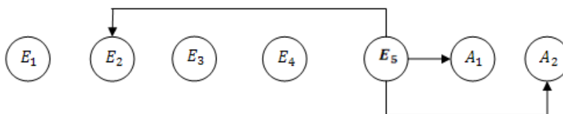
Рис. 5. Граф для индикатора E_5
