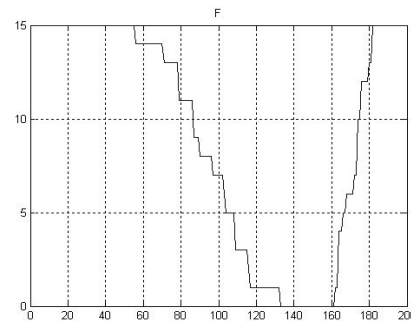
Рис. 2. Значения F(c_0)
