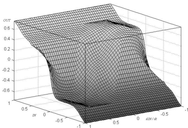
Рис. 2. Поверхность отклика OUT = f(IN, dIN / dt)
