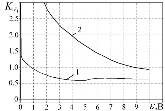
Рис. 4. Зависимости коэффициента передачи нечеткого регулятора по ошибке:
