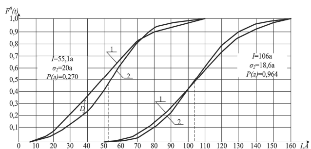
Рис. 3. Упорядоченные диаграммы нагрузки тяговых двигателей рудничных электровозов при движении с груженым и порожняковым составом (а) и при погрузочно-разгрузочных режимах (б)
