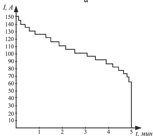
Рис. 3. Упорядоченные диаграммы нагрузки тяговых двигателей рудничных электровозов при движении с груженым и порожняковым составом (а) и при погрузочно-разгрузочных режимах (б)
